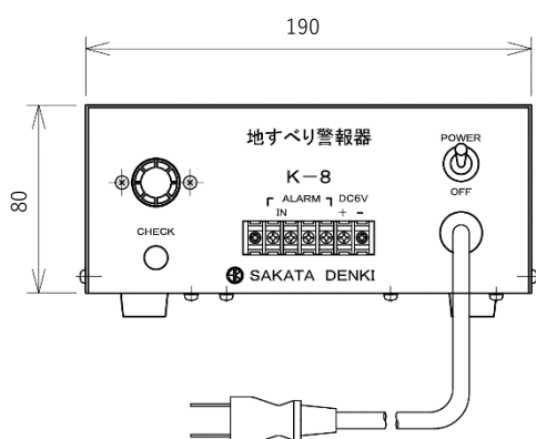
形状寸法 K-8
