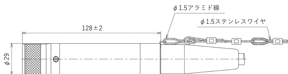
形状寸法
